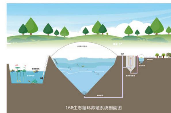
图1 漏斗形池塘剖面图（效果图）
