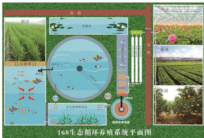
图2 漏斗形池塘生态循环系统平面图
