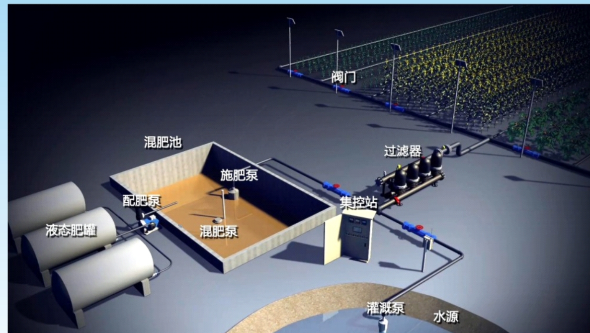
智能水肥一体化系统展示图
