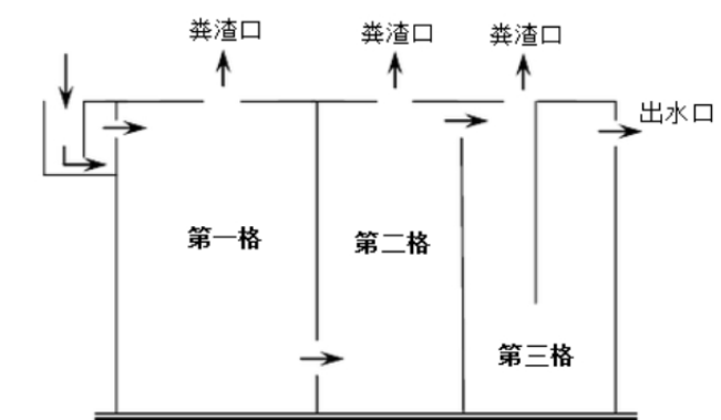
图1-2 典型三格式化粪池示意图
